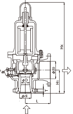
AF-4M (开放式, 不带扳手)
