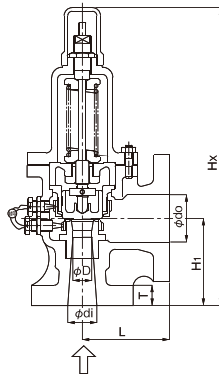
AF-4M (开放式, 不带扳手)
